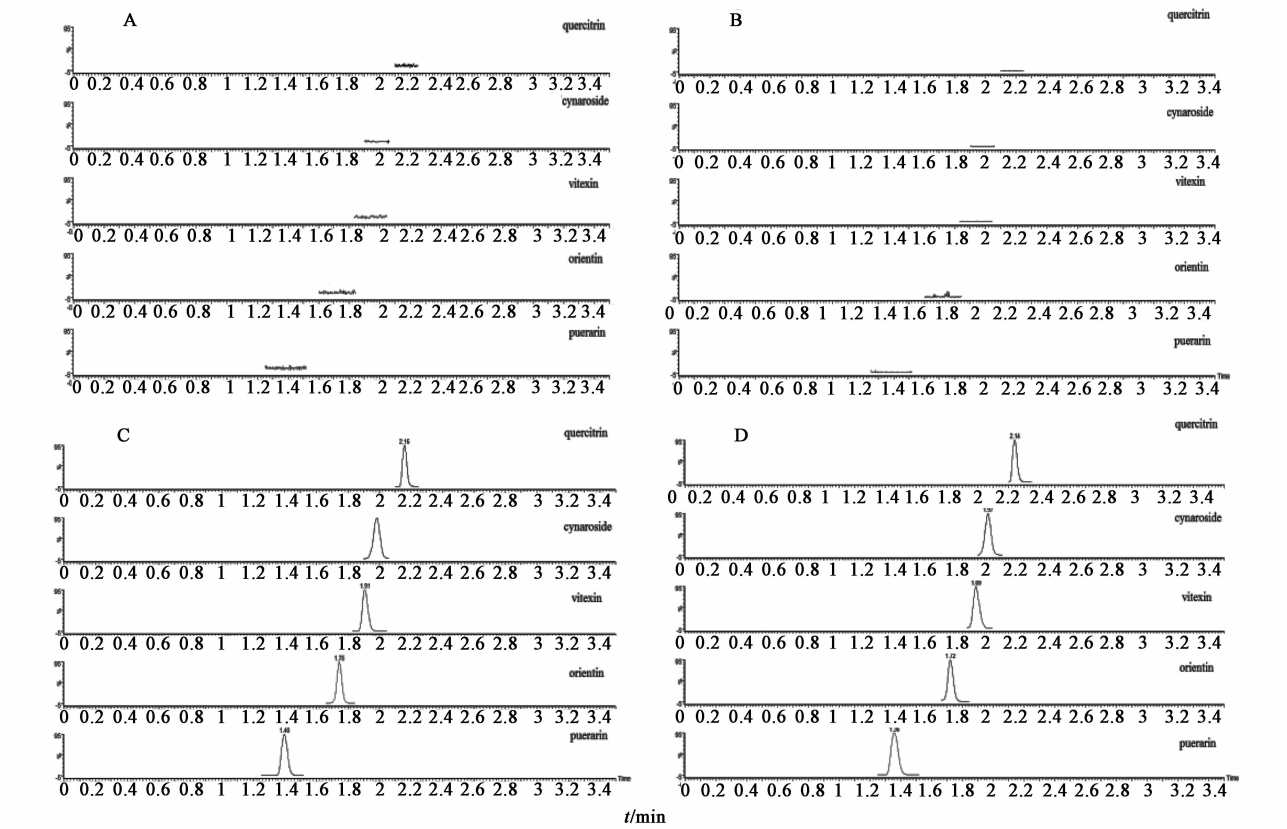
A. 空白血浆;B. 空白缓冲液;C. 血浆样品;D. 缓冲液样品 图 1 荭草素、牡荆素、木犀草苷、槲皮苷及内标在空白血浆及缓冲液中的流动色谱
